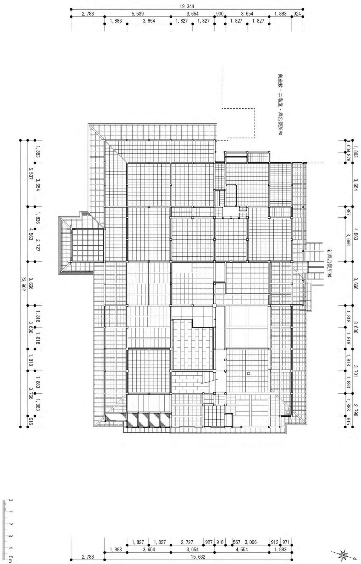
第 11 図、修理前 見上図
